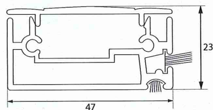
Doorsnede:
