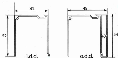
U-profiel (bovengeleider)
