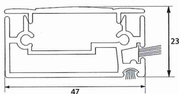
Doorsnede:
