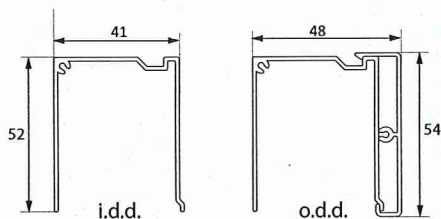
U-profiel (bovengeleider)
