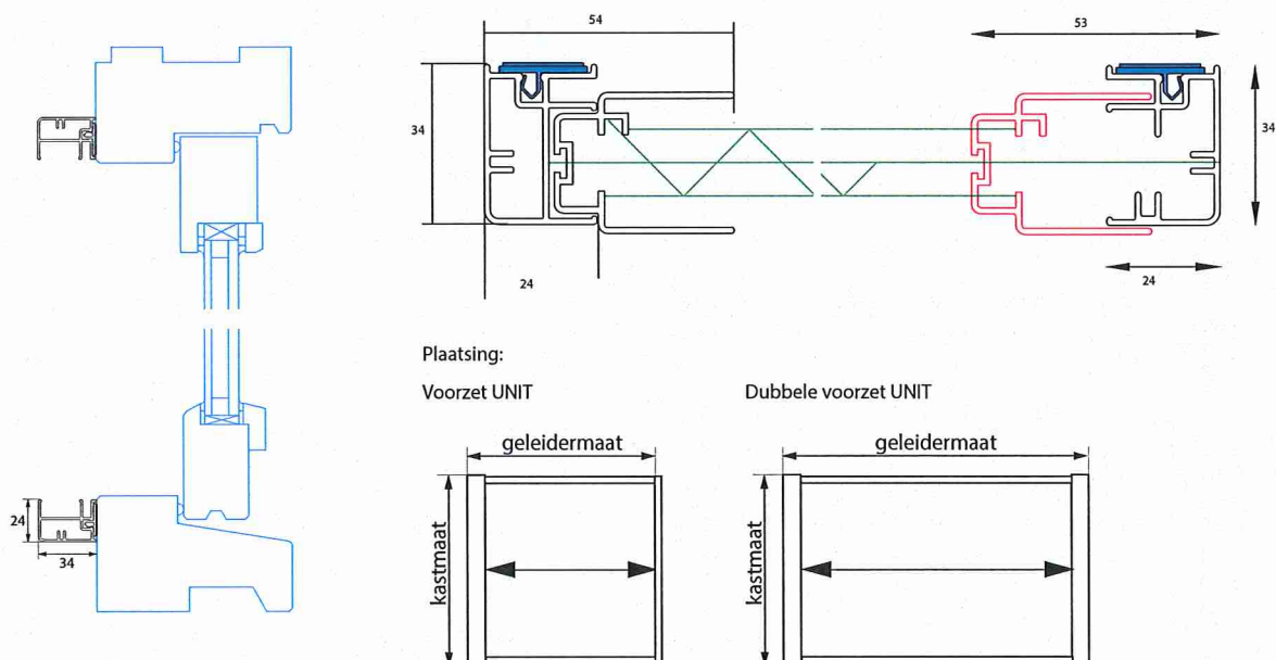
Doorsnede:
