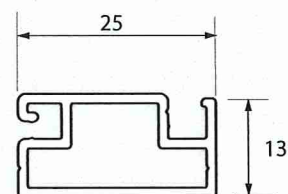
Doorsnede:
