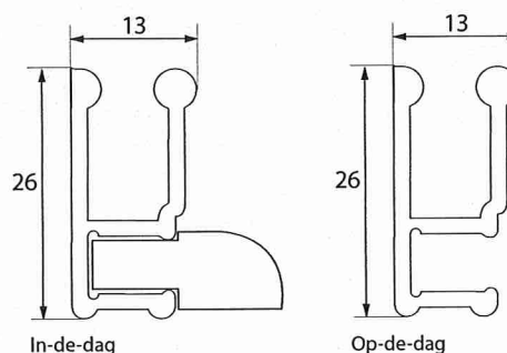
Doorsnede:
