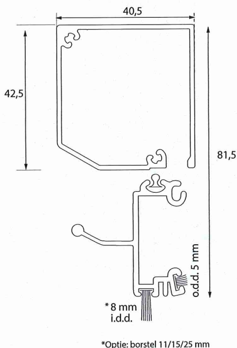
Doorsnede:
