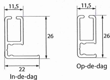
Doorsnede:
